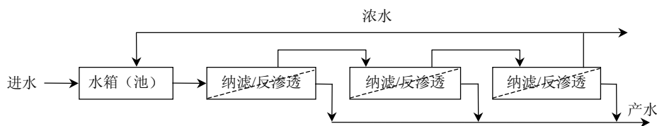
图 4 一级多段循环式系统基本工艺流程图
