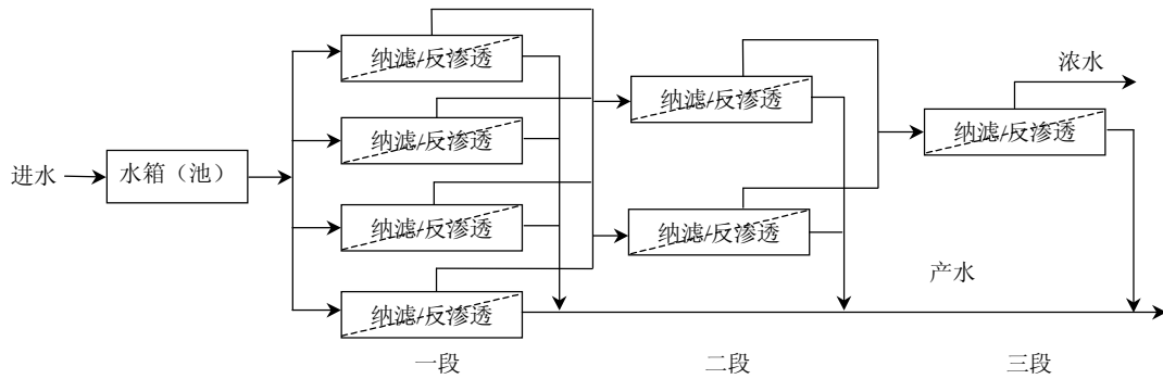
图6 一级多段系统基本工艺流程图
