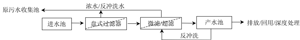
图 1 微滤、超滤系统基本工艺流程图
