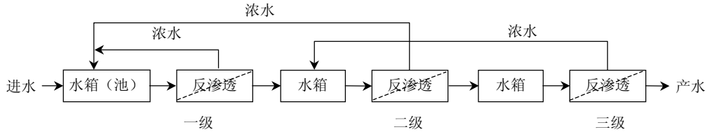
图7 多级系统基本工艺流程图
