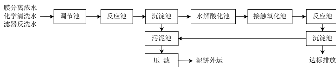
图 8 浓水处理基本工艺流程图
