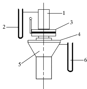
图2 流量检测系统示意
