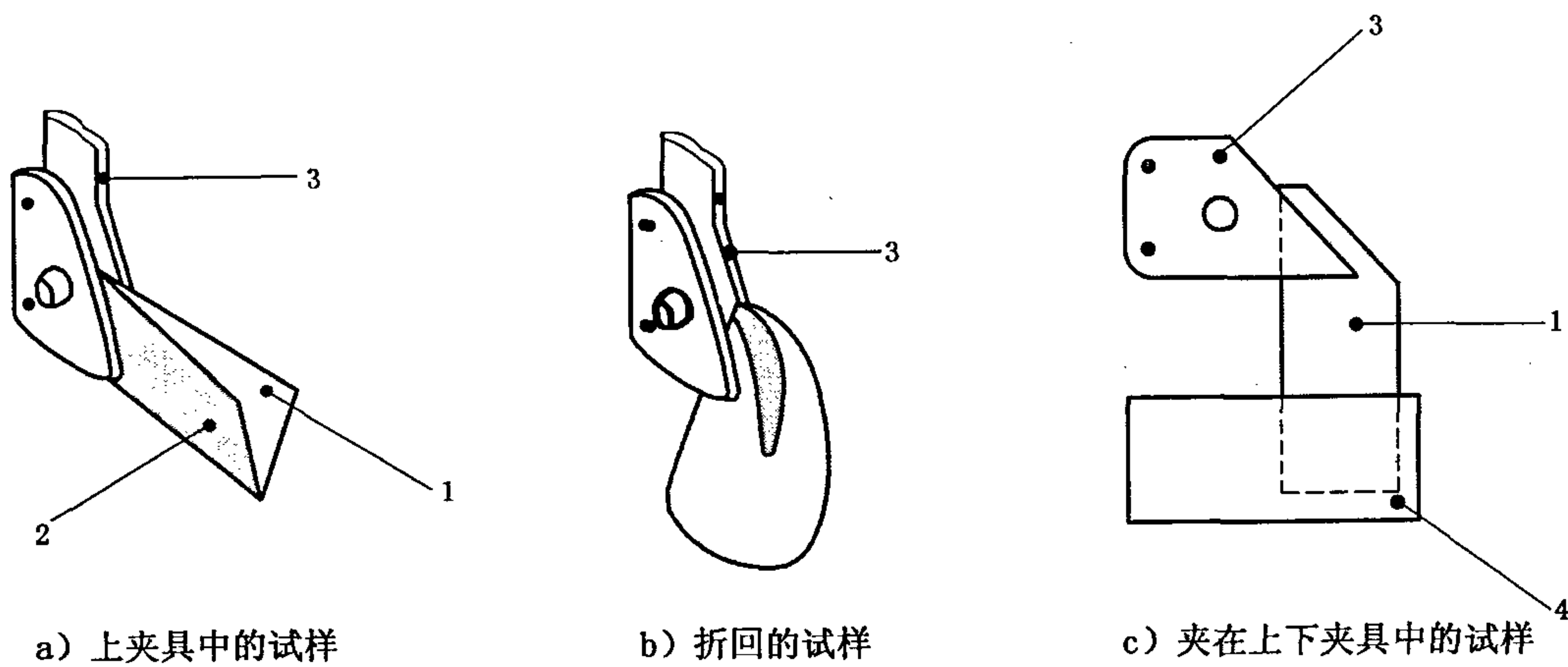
图 44 上夹具
