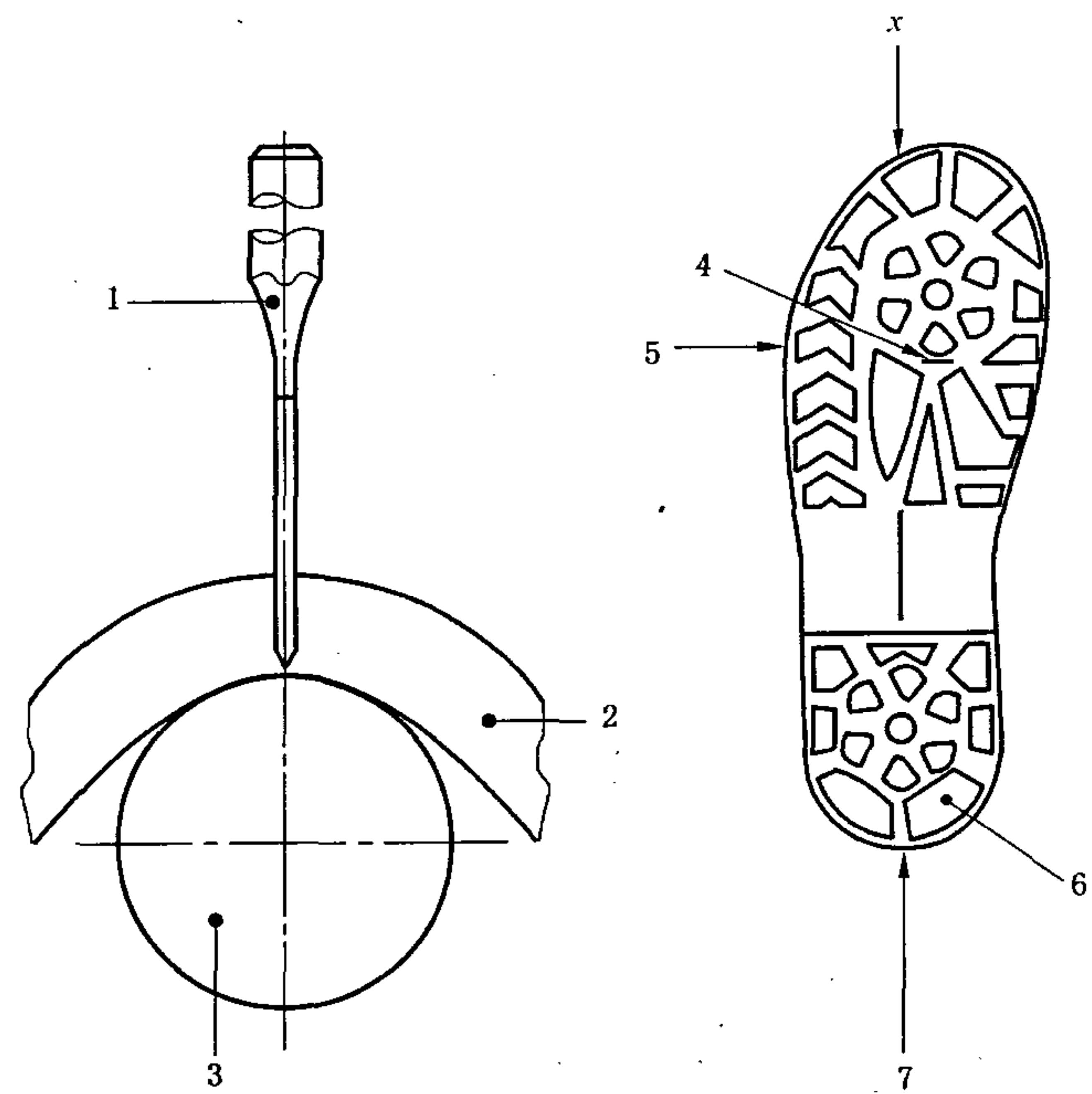
图 58 割口刀
