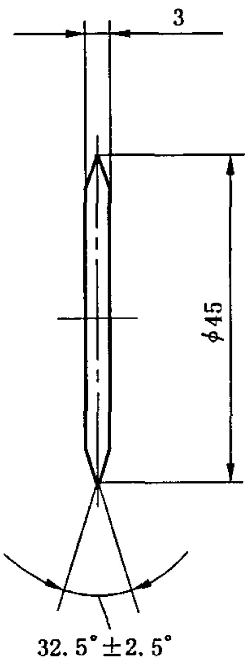
图 48 圆刀片规格
