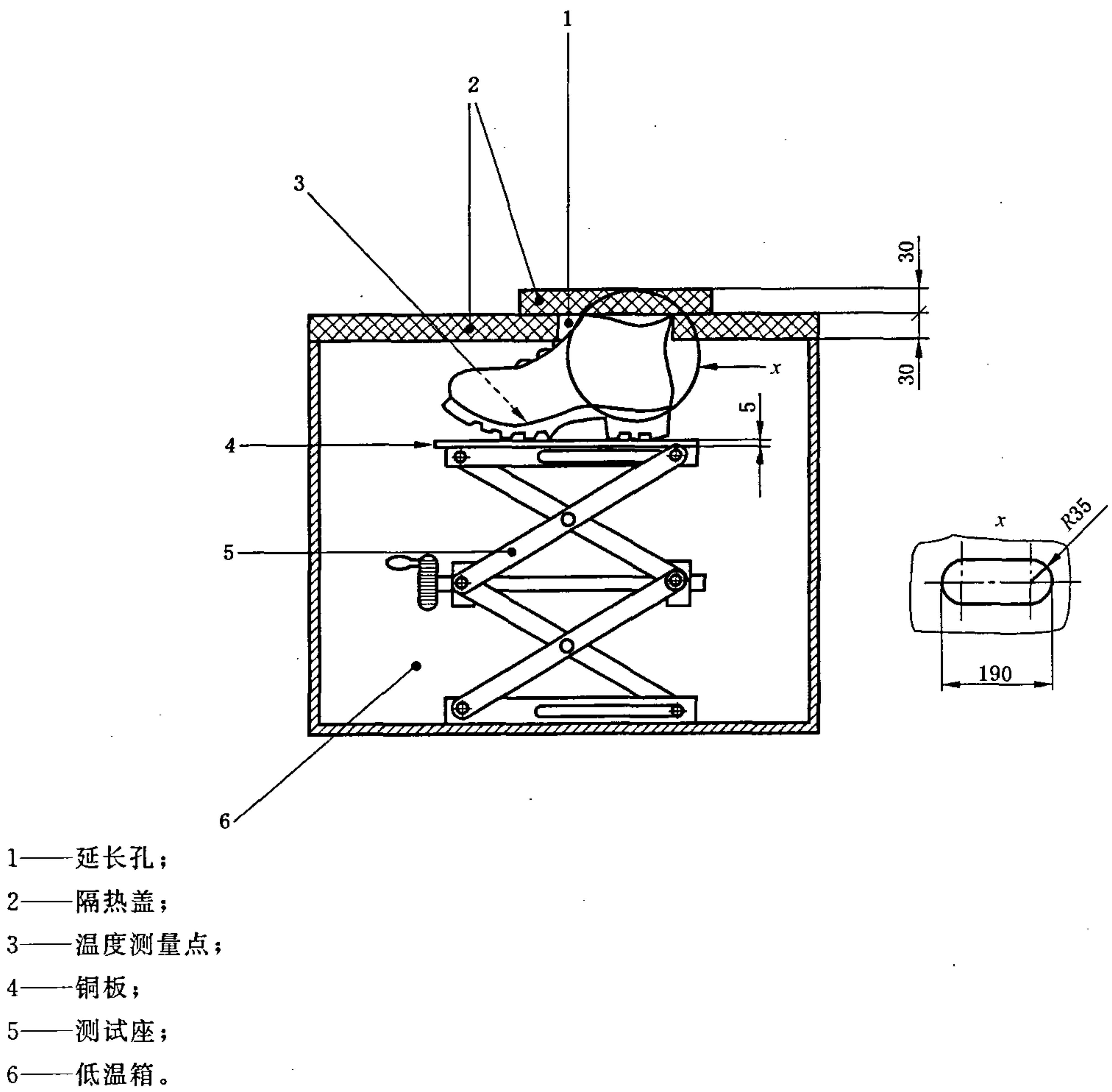
图 22 防寒性测试装置
