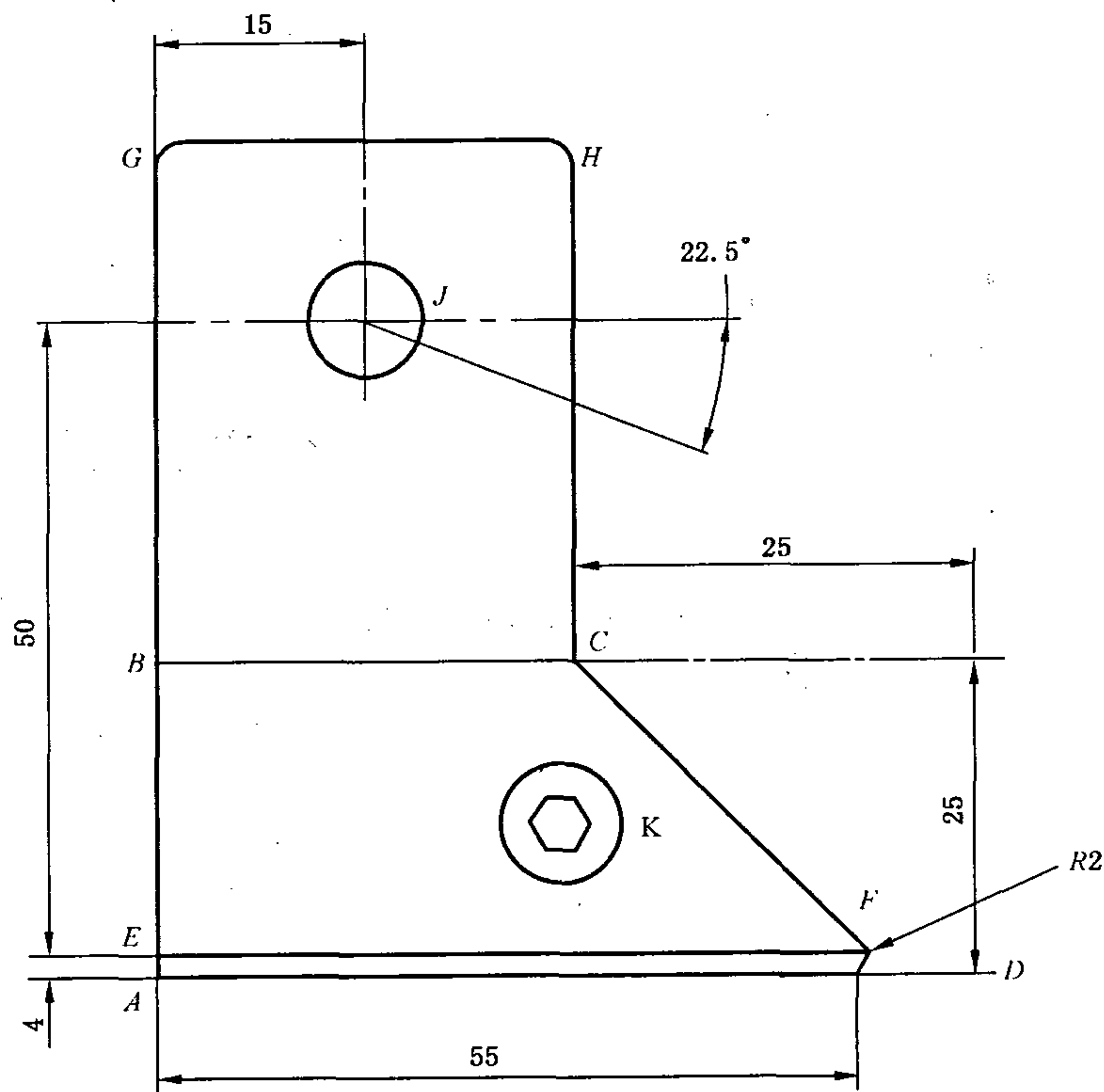
图 44 上夹具
