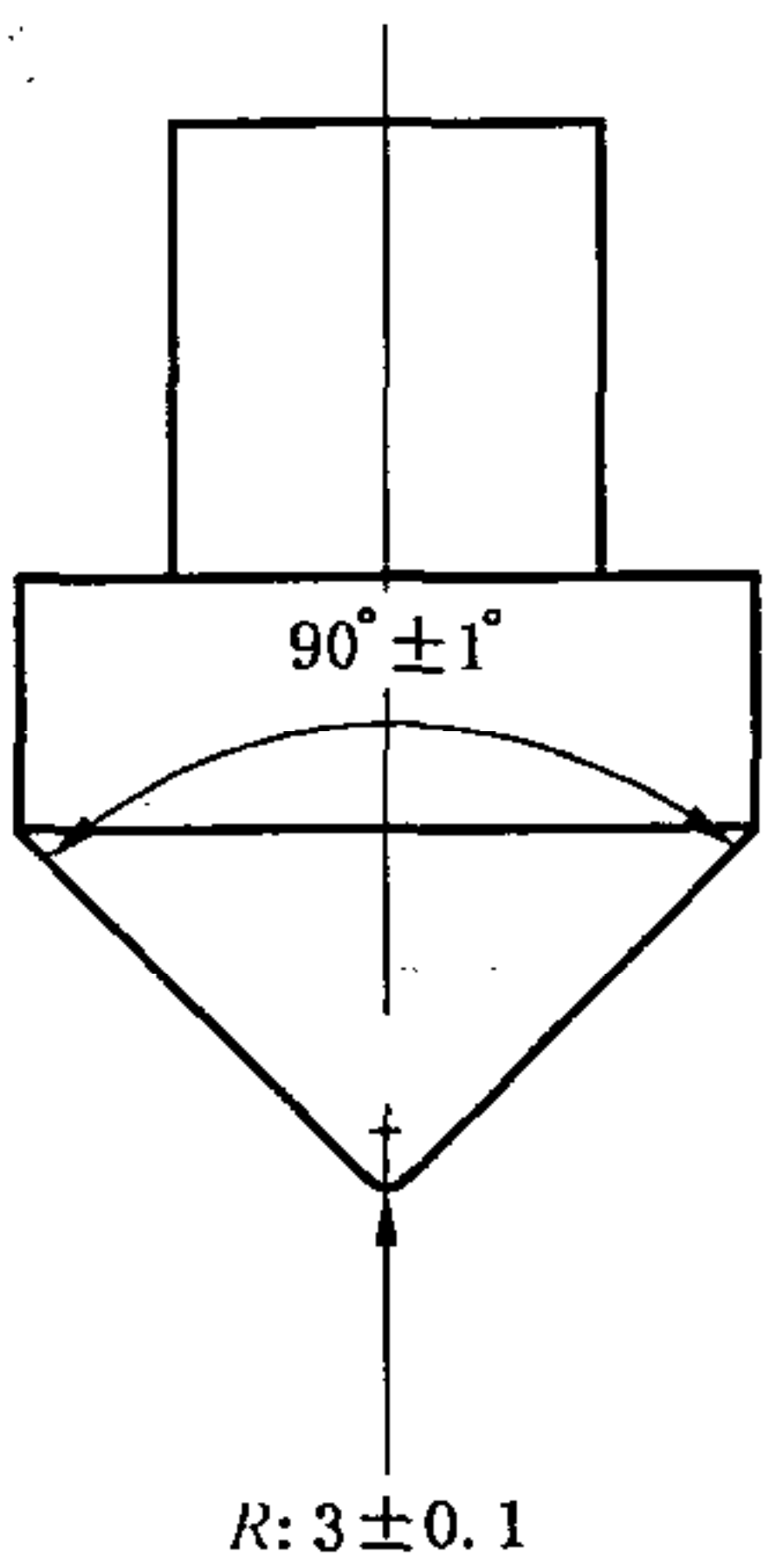
图 9 冲击锤
